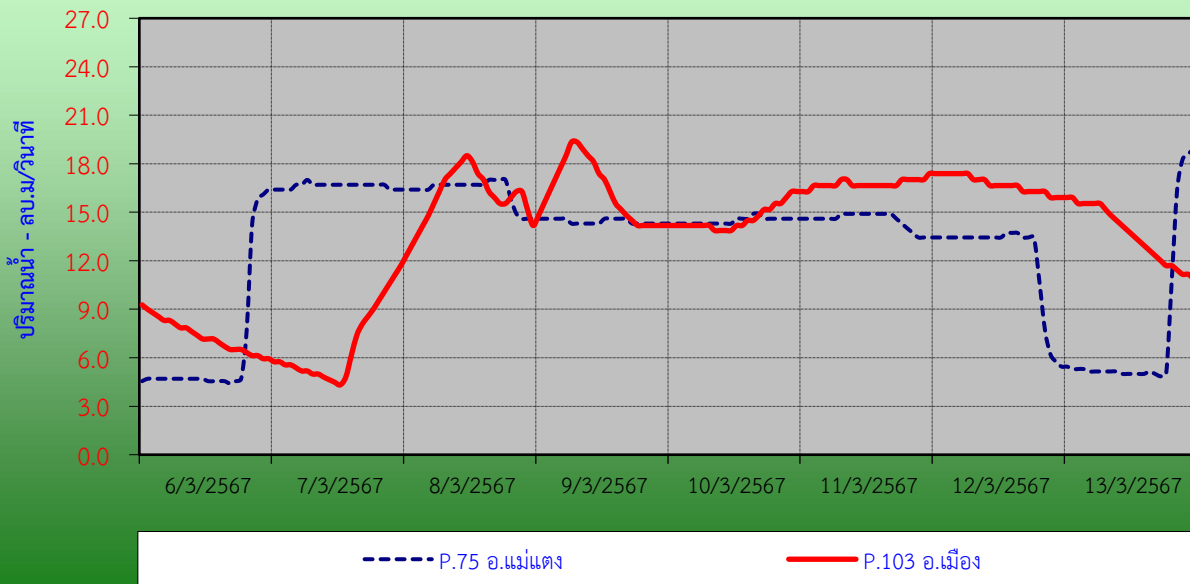
กราฟแสดงปริมาณน้ำปิ้งรายชั่วโมงรอบวันที่ 10/2567 ที่สถานีแม่ น้ำปิ้ง ( P.75) บ้านซ้อแล อ.แม่แตง และที่สถานีแม่ น้ำปิ้ง ( P.103) บ้านป่าข่อยใต้ อ.เมือง จ.เชียงใหม่
